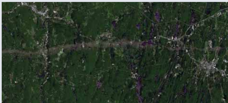
Huella de un tornado cerca de Sturbridge, Massachusetts. EEUU
