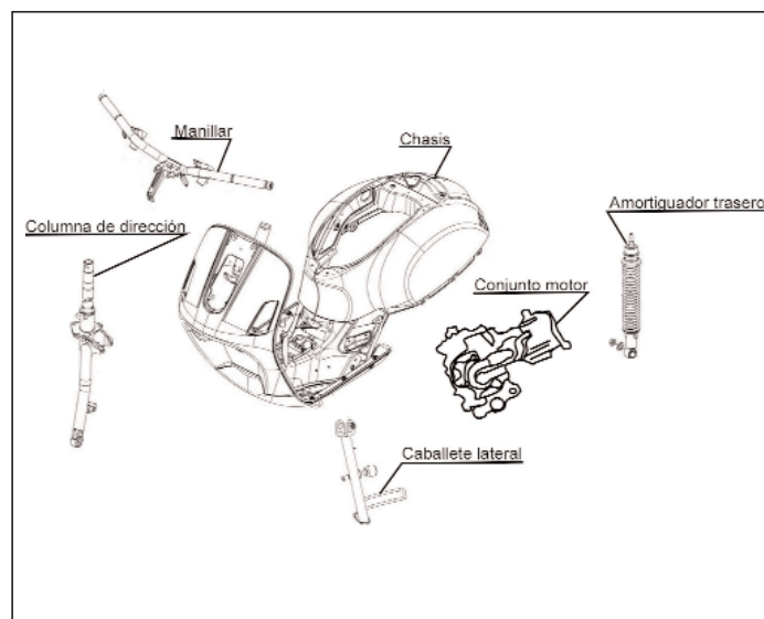
Figura 1.- Unión del chasis
