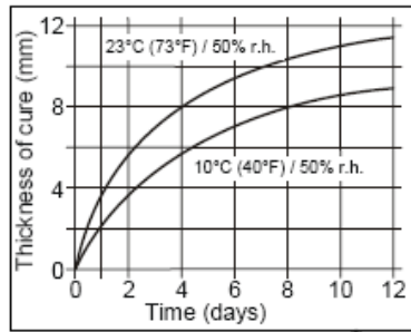
Diagrama 1: Velocidad de curado Sikaflex®-529AT
