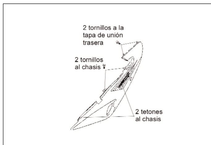
Figura 6.- Unión de la tapa trasera
