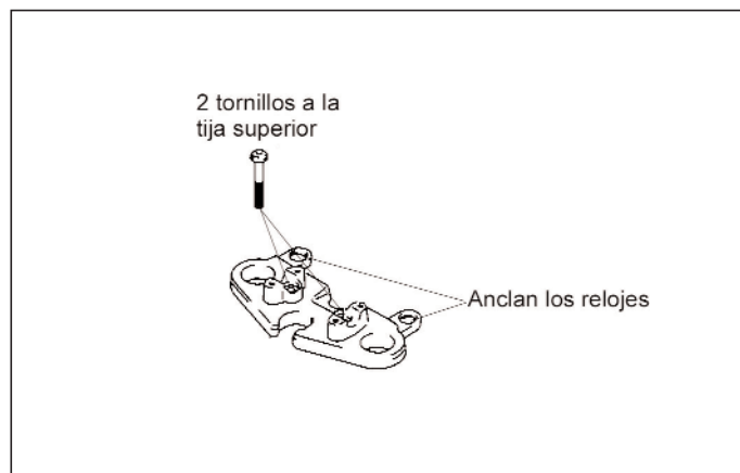
Figura 21.- Unión del soporte de manillar
