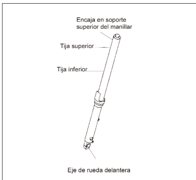
Figura 20.- Unión de la barra de suspensión
