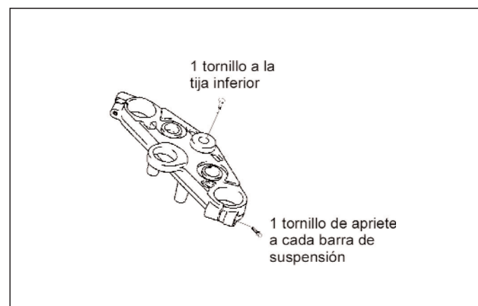
Figura 22.- Unión de la tija superior
