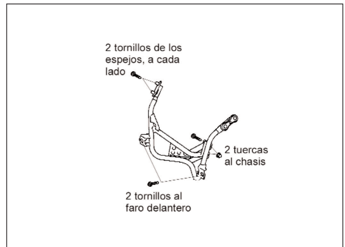
Figura 27.- Unión de la araña
