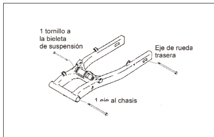
Figura 13.- Unión del basculante
