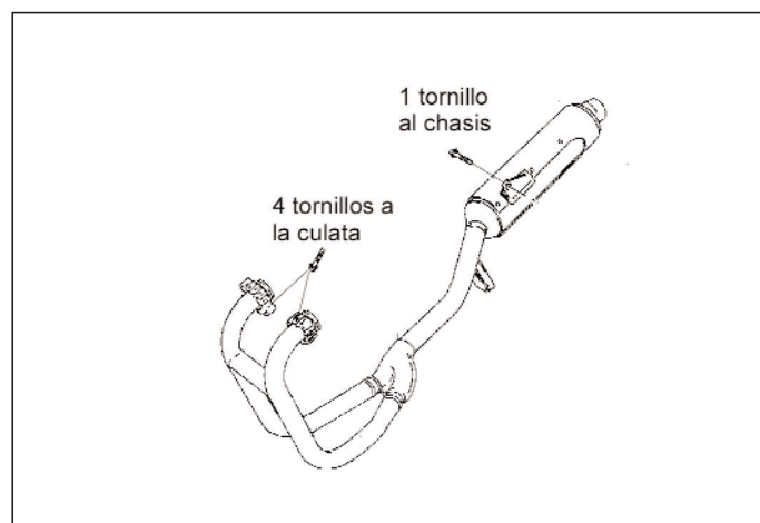
Figura 14.- Unión del escape
