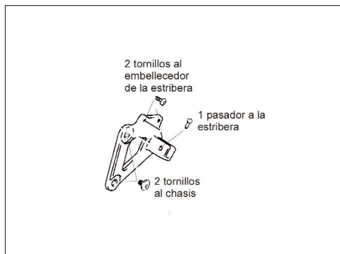
Figura 3.- Unión de la estribera de conductor
