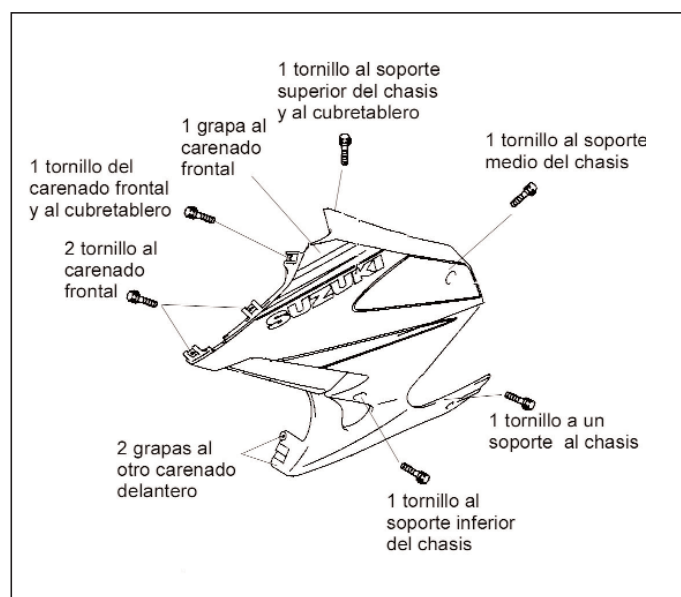
Figura 9.- Unión del carenado delantero
