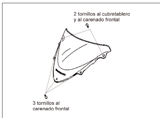
Figura 26.- Unión de la cúpula
