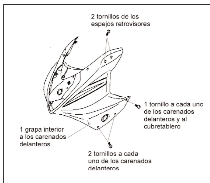
Figura 24.- Unión del carenado frontal
