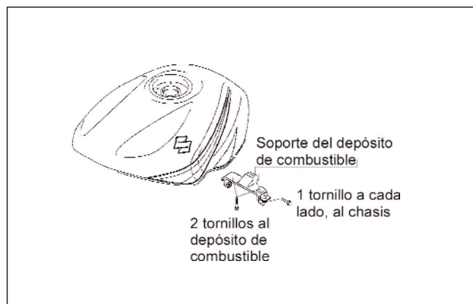
Figura 15.- Unión del depósito de combustible
