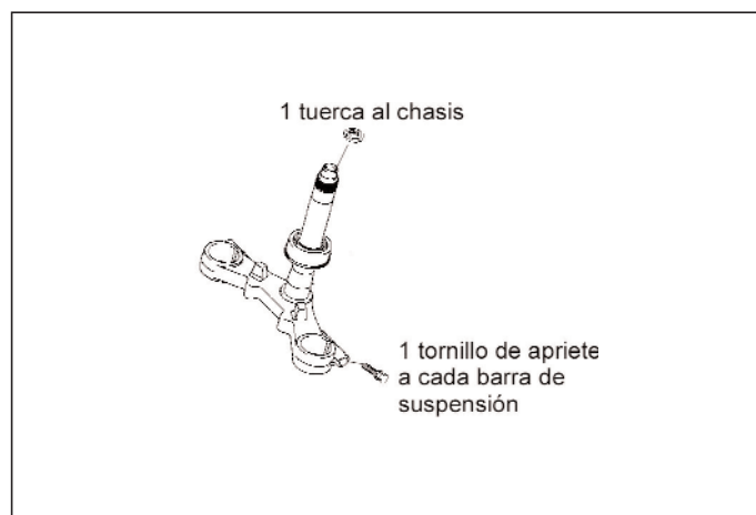
Figura 23.- Unión de la tija inferior
