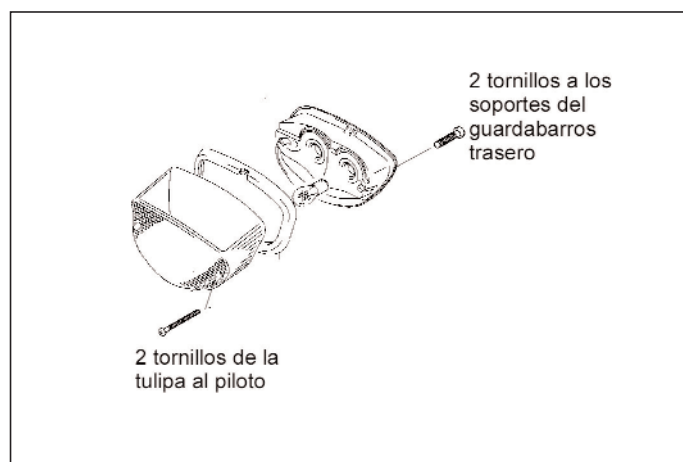
Figura 8.- Unión del piloto trasero
