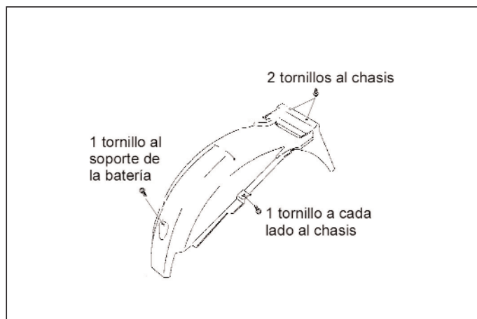
Figura 9.- Unión del guardabarros trasero
