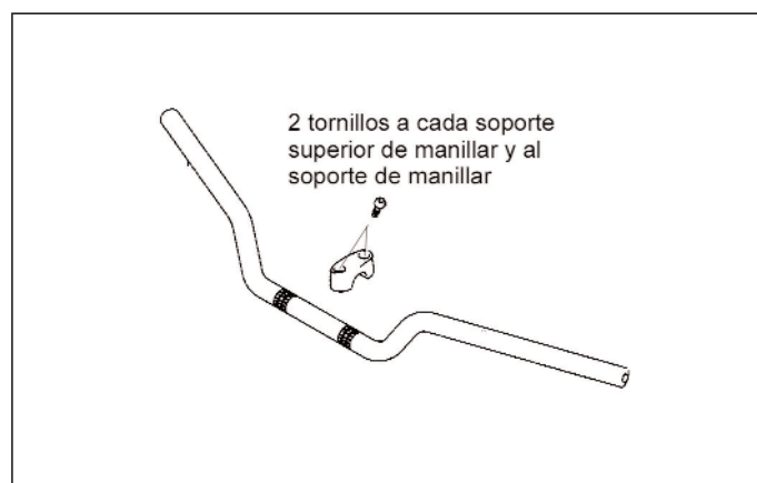
Figura 16.- Unión del manillar
