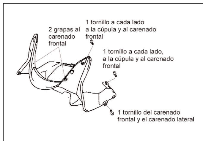
Figura 18.- Unión de la tapa cubretablero
