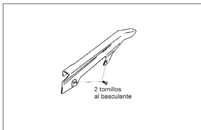
Figura 4.- Unión del cubrecadenas
