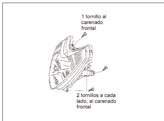
Figura 25.- Unión del faro delantero
