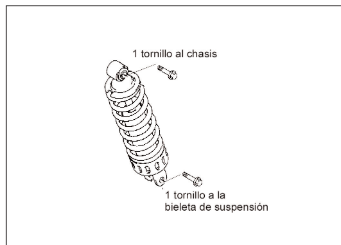
Figura 12.- Unión del amortiguador trasero
